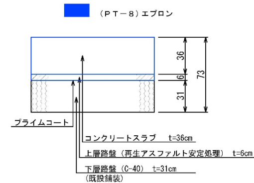
舗装構成図
