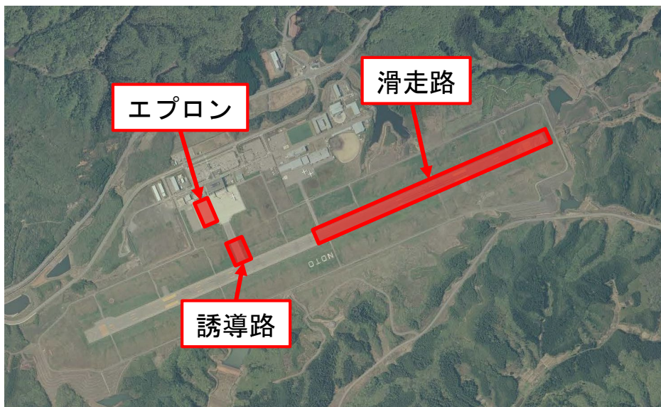
滑走路
