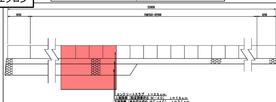
エプロン
