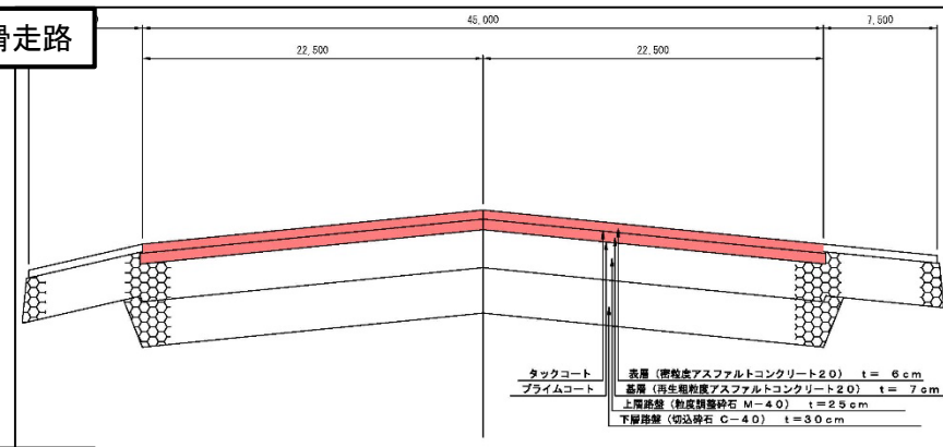
誘導路
