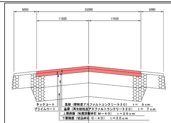
エプロン
